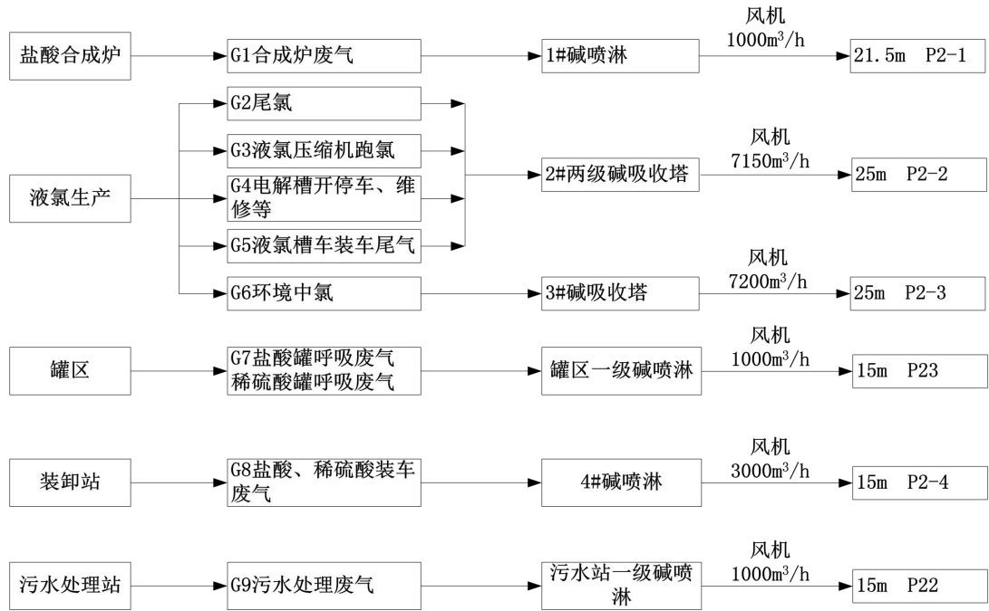
图 2.3-11 本项目废气收集走向图 (1)
