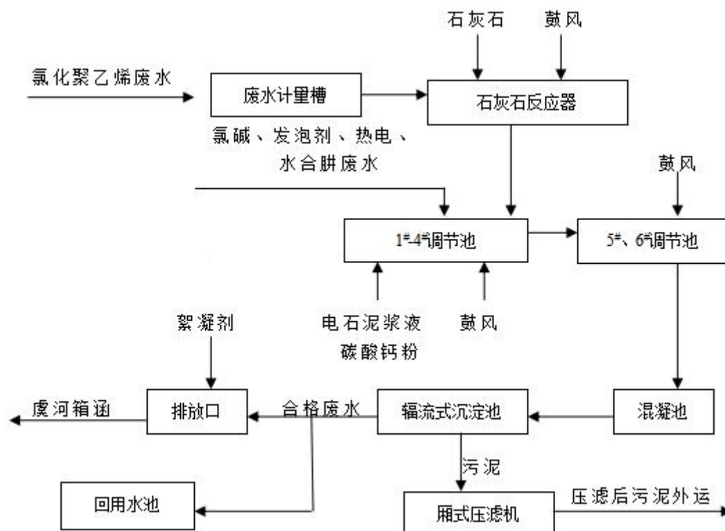
图 2.1-7 老厂区现有污水处理站工艺流程图
