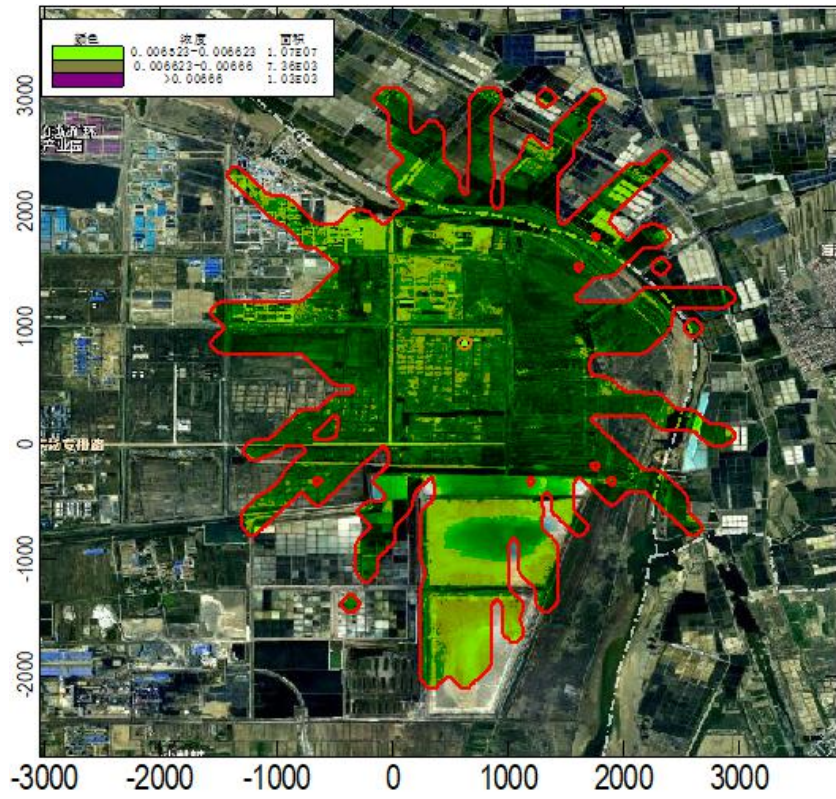
图 4.2-5 拟建项目硫化氢区域网格点最大小时浓度分布图 ( \text{mg}/\text{m}^3 )
