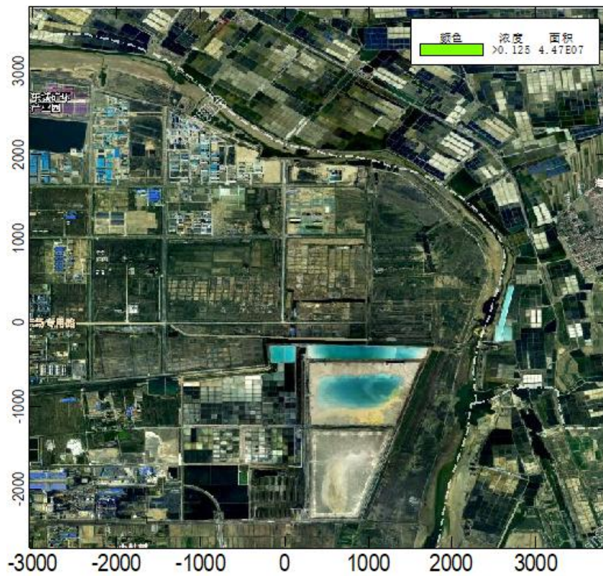
图 4.2-4 拟建项目氨区域网格点最大小时浓度分布图 ( \text{mg}/\text{m}^3 )
