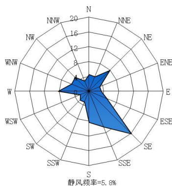
图 4.2-1 昌邑近 20 年（1998~2017 年）风向频率玫瑰图
