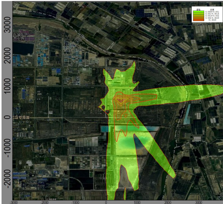
图 4.2-3 拟建项目氯化氢区域网格点最大小时浓度分布图 ( \text{mg}/\text{m}^3 )
