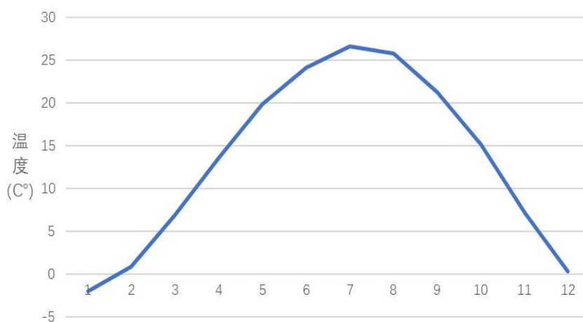
图 4.2-2 昌邑近 20 年年平均温度月变化曲线
