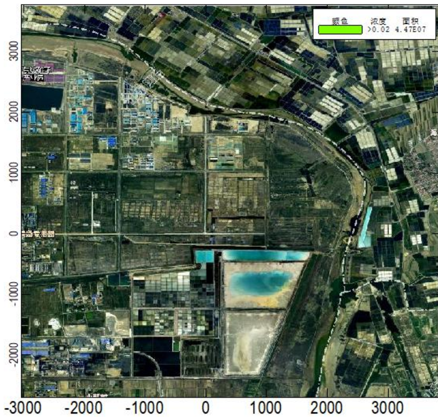
图 4.2-6 拟建项目硫酸雾区域网格点最大小时浓度分布图 ( \text{mg}/\text{m}^3 )
