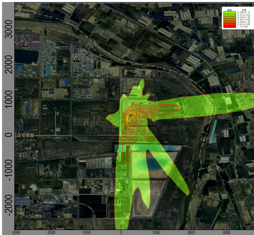
图 4.2-2 拟建项目氯区域网格点最大小时浓度分布图 ( \text{mg}/\text{m}^3 )
