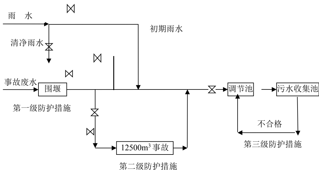
图 5.6-9 事故废水截流、收集及处理的系统操作图
