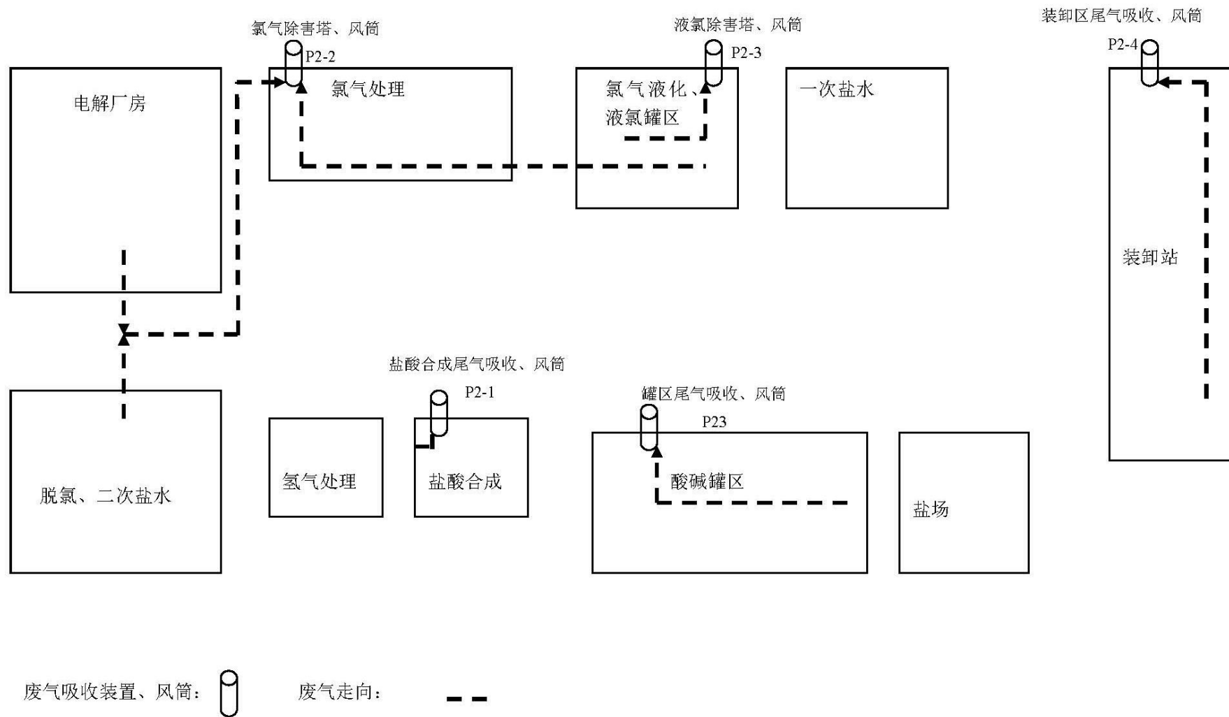
图 2.3-11 本项目废气收集走向图 (2)
